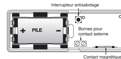
Détecteur de basse température Vue arrière
